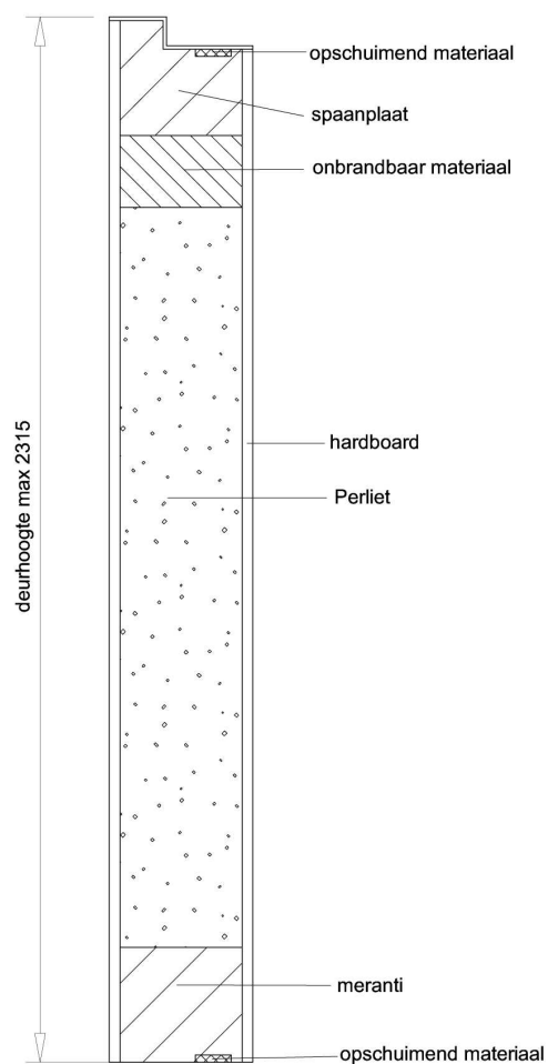
Doorsnede BB
