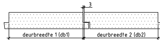
Doorsnede AA
