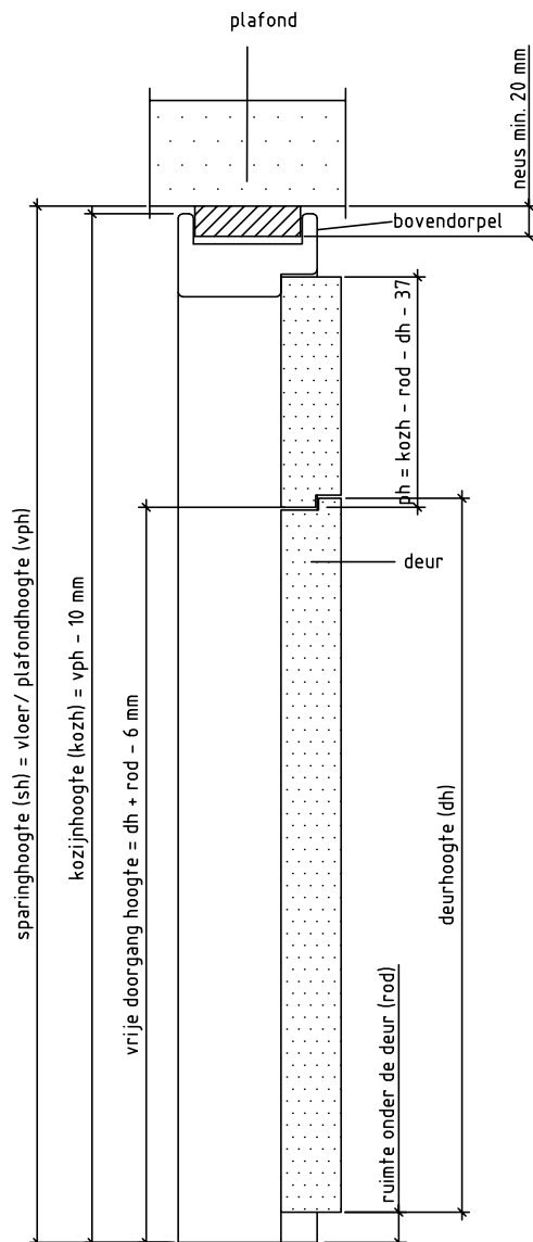
Doorsnede BB
