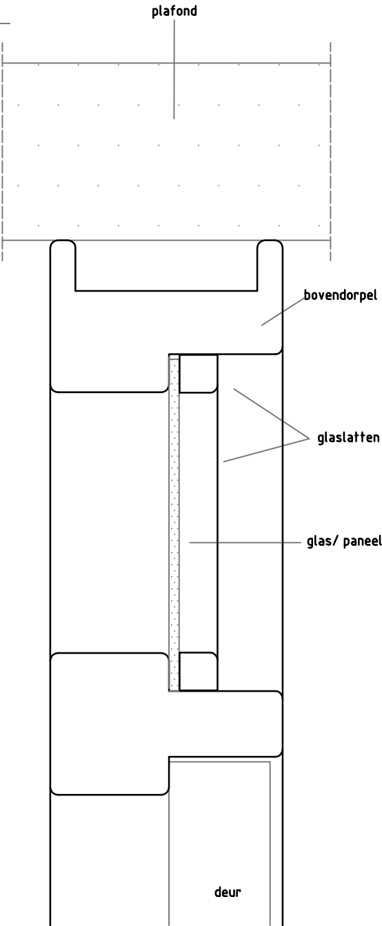
Detail 2: bovendorpel
