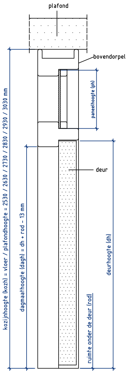
Doorsnede BB
