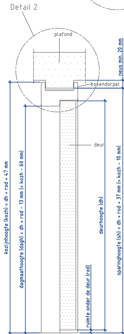
Doorsnede BB
