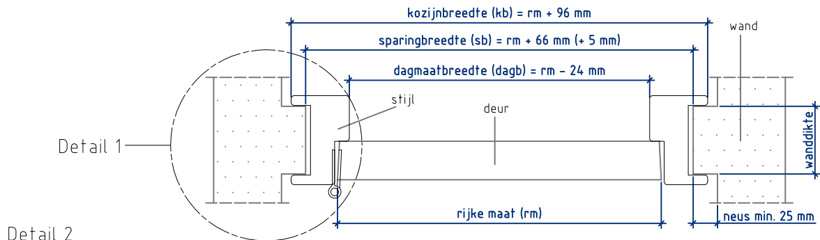
Doorsnede AA
