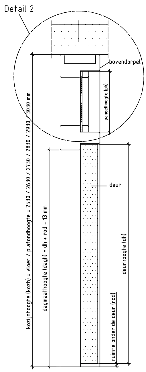
Doorsnede BB
