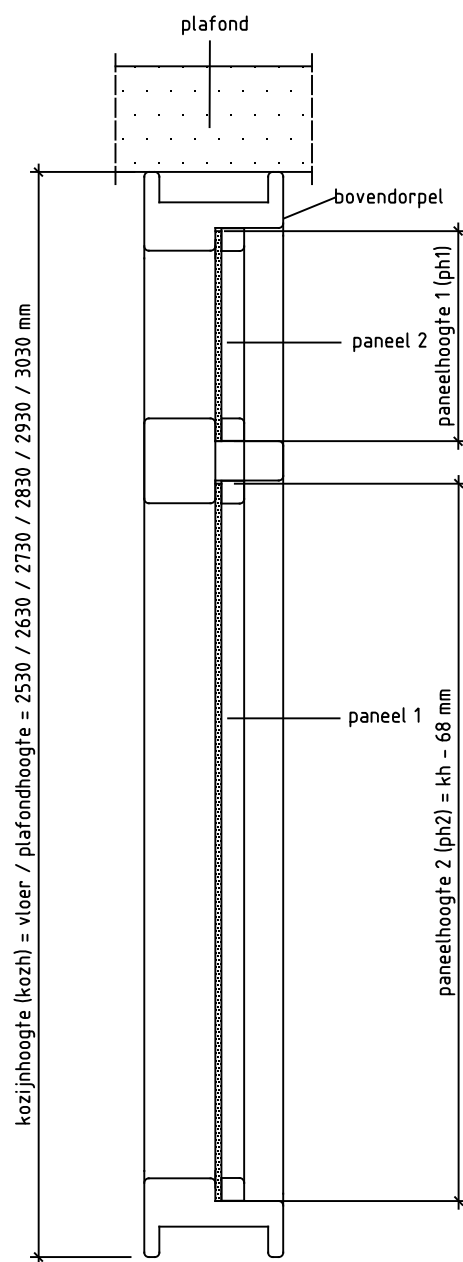
Doorsnede CC
