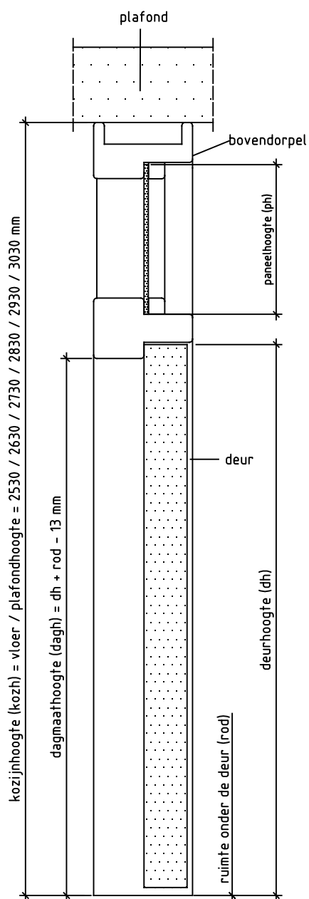
Doorsnede BB
