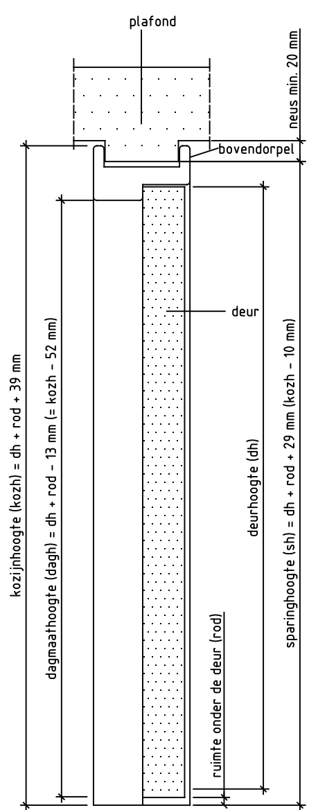
Doorsnede BB
