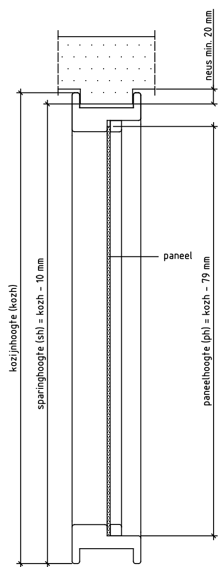
Doorsnede CC
