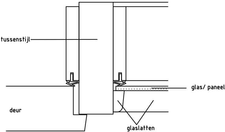
Detail 5: tussenstijl
