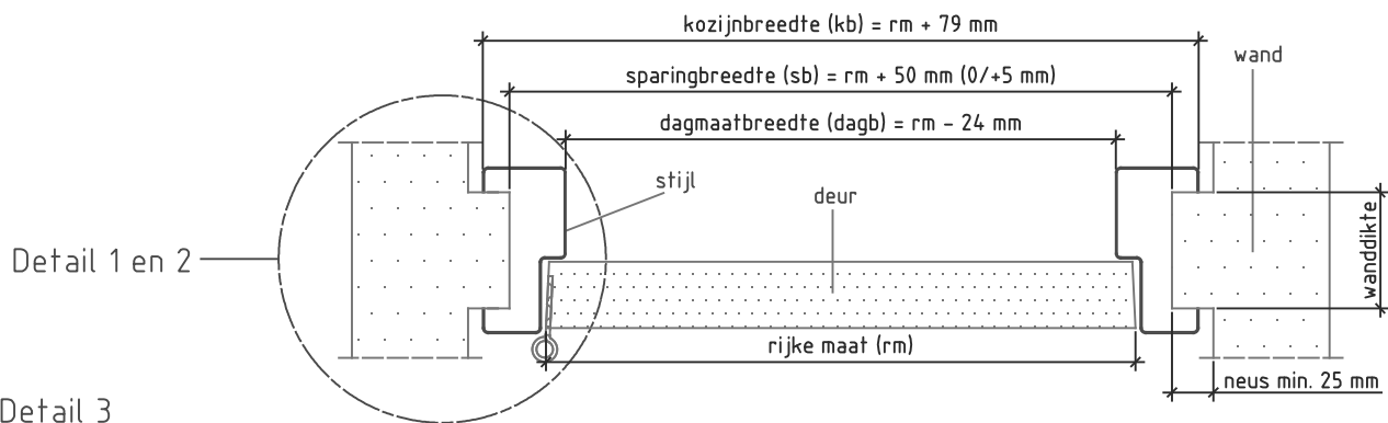
Doorsnede AA
