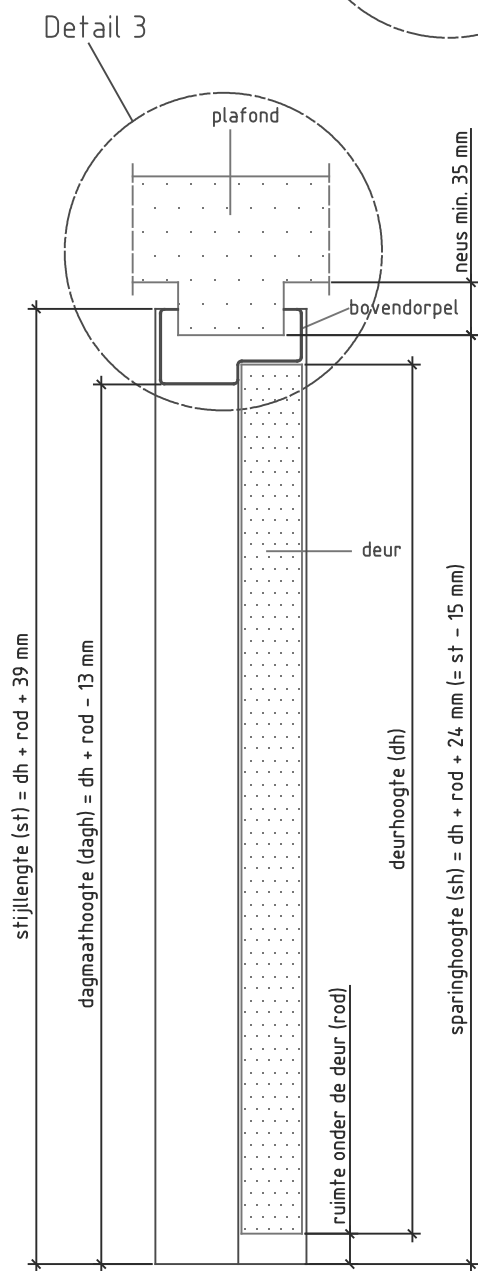
Doorsnede BB
