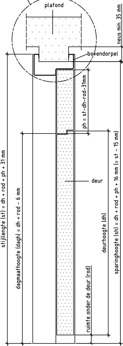
Doorsnede BB
