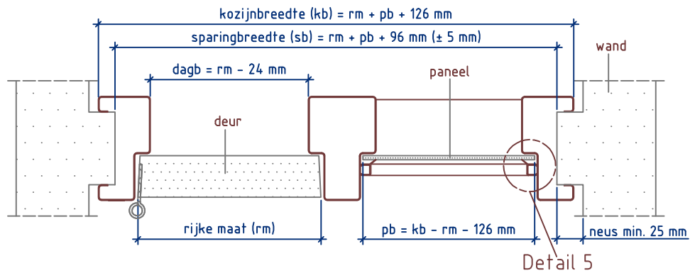
Doorsnede AA
