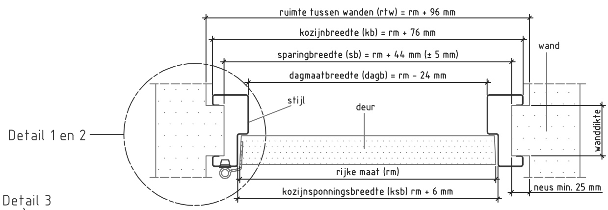
Doorsnede AA
