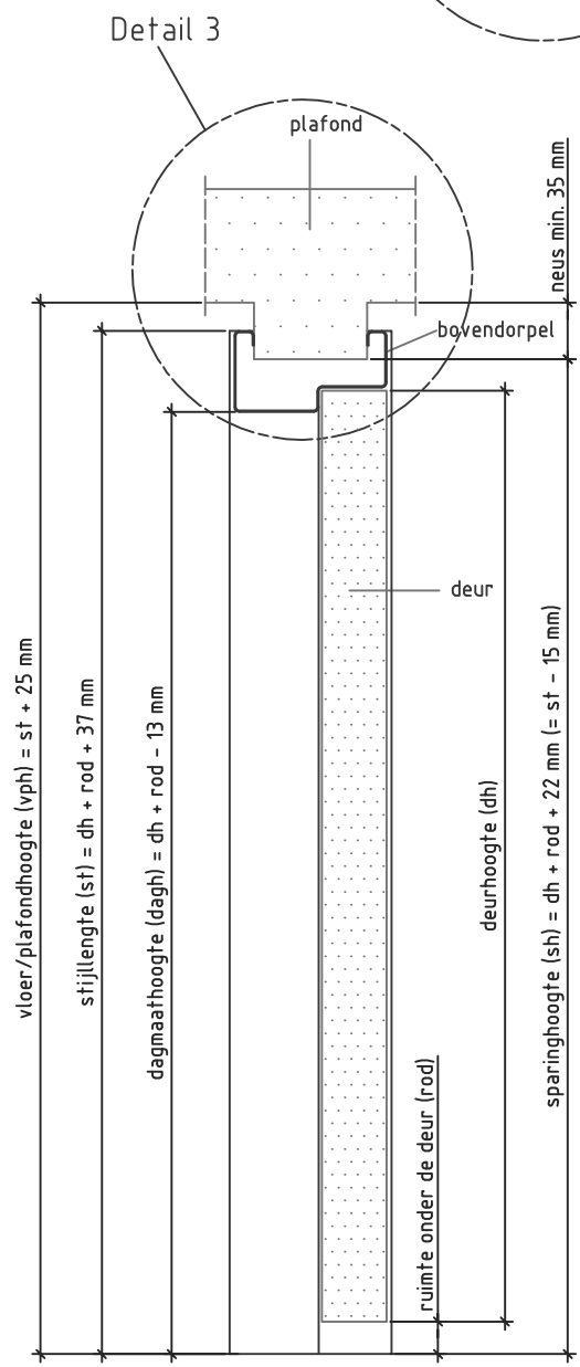
Doorsnede BB
