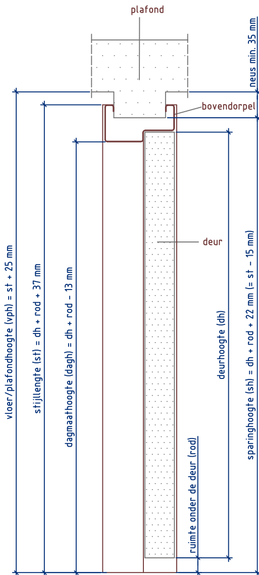
Doorsnede BB
