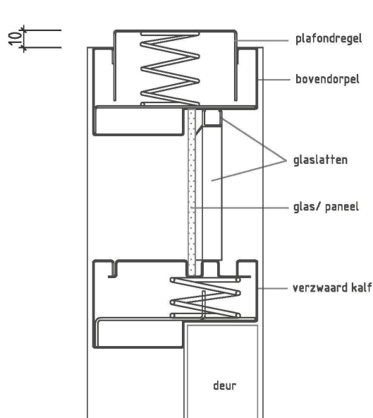
Plafondregel in "gespannen" toestand (bij levering)
