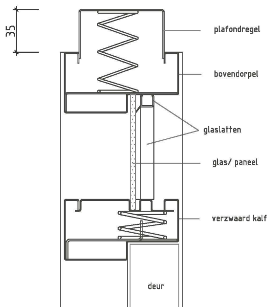
Plafondregel maximaal (gemonteerd)
