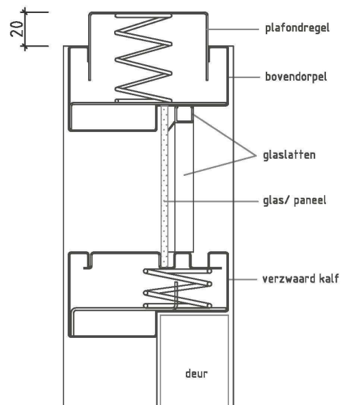
Plafondregel minimaal (gemonteerd)
