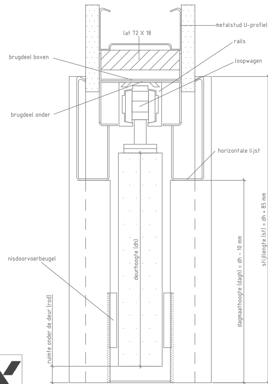
Doorsnede AA
