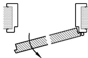
Rechtsdraaiende deur, constructieprincipe
