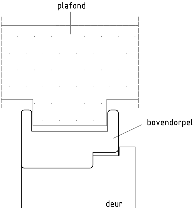
Detail 2: bovendorpel
