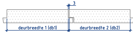
Doorsnede AA
