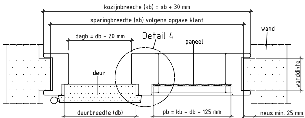
Doorsnede AA
