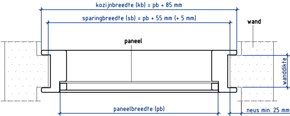
Doorsnede AA
