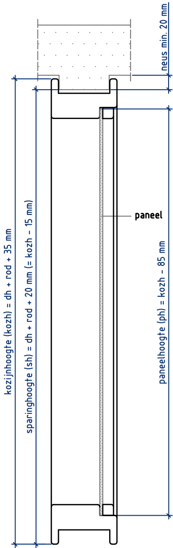
Doorsnede BB
