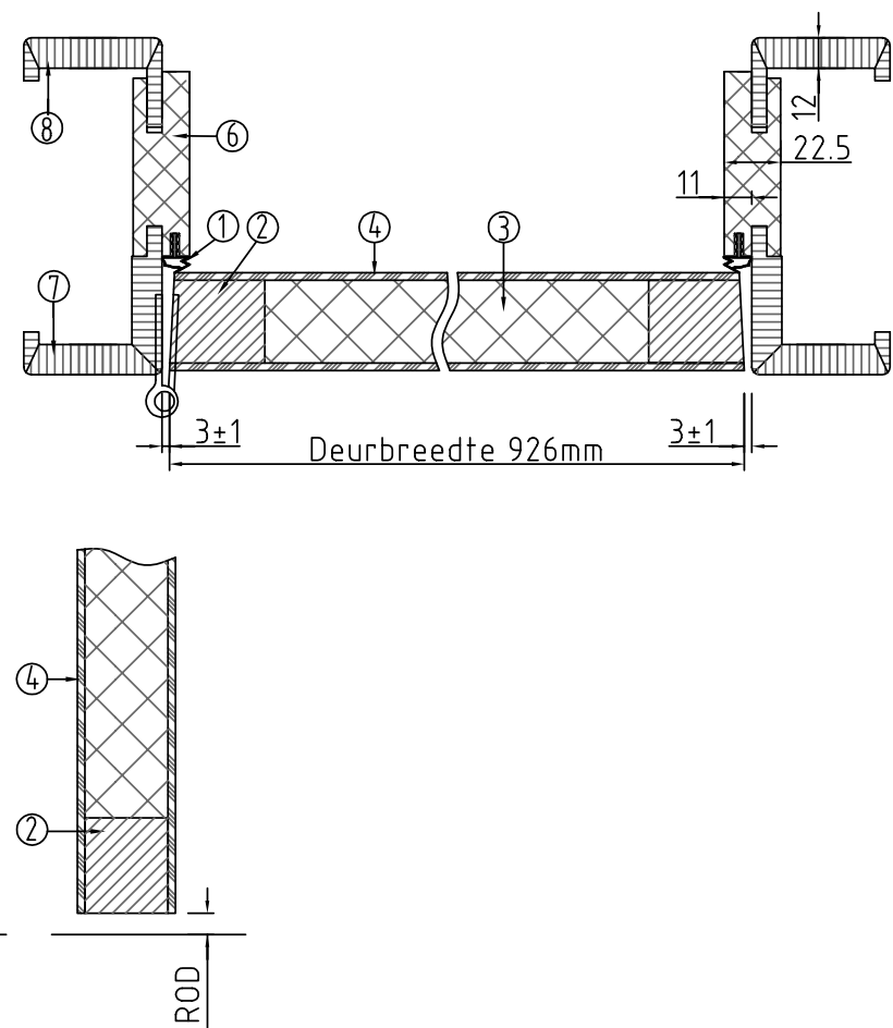
Doorsnede BB
