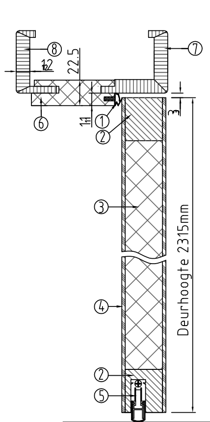
Doorsnede AA
