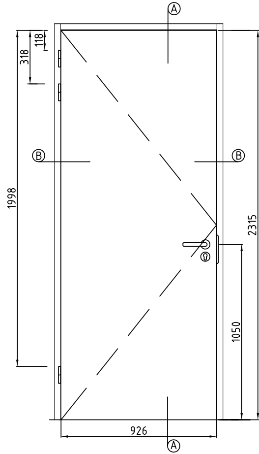
Vooraanzicht
