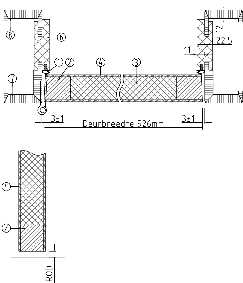
Doorsnede BB
