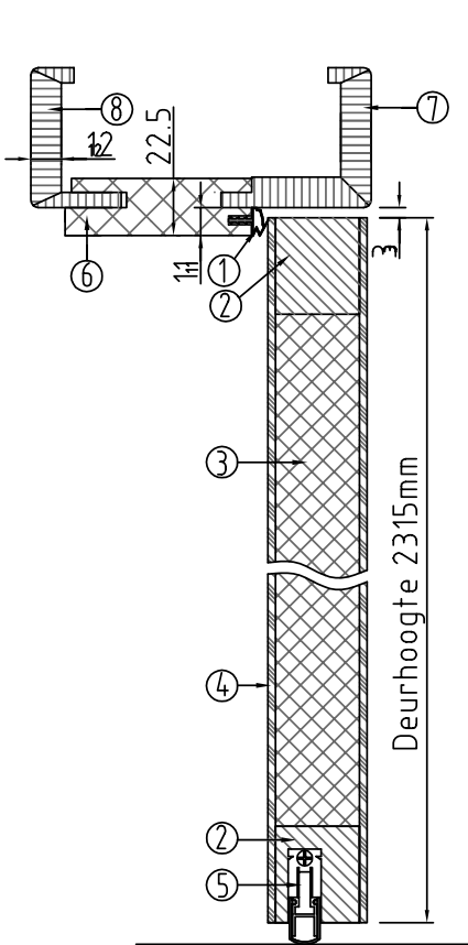
Doorsnede AA
