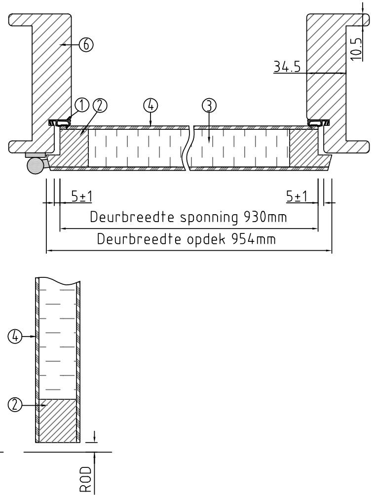
Doorsnede BB
