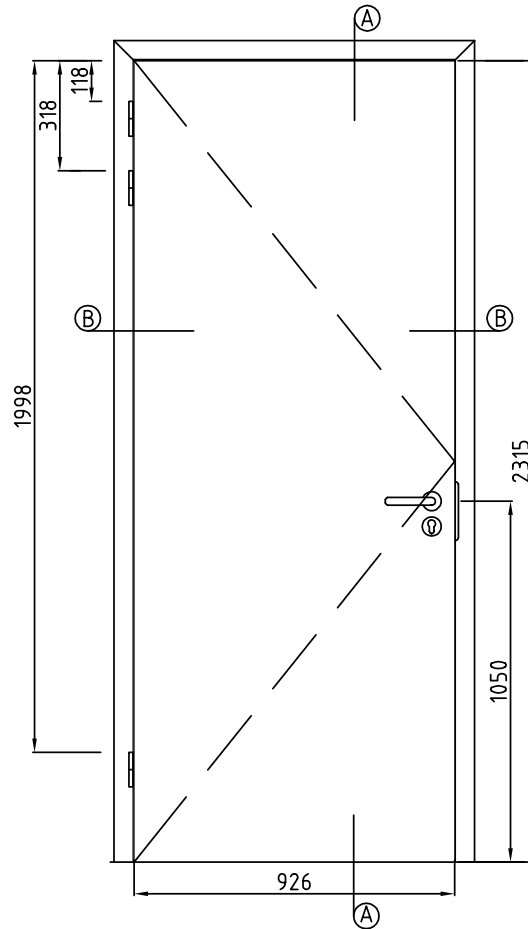
Vooraanzicht
