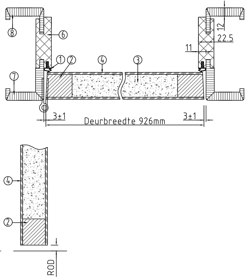
Doorsnede BB
