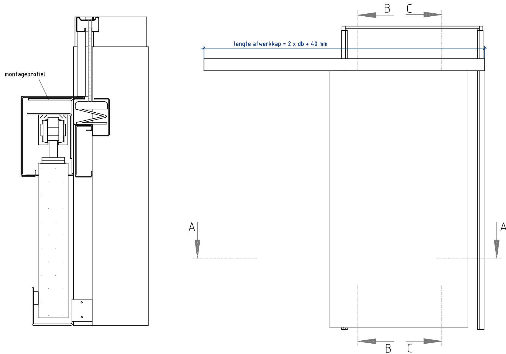
Doorsnede BB
