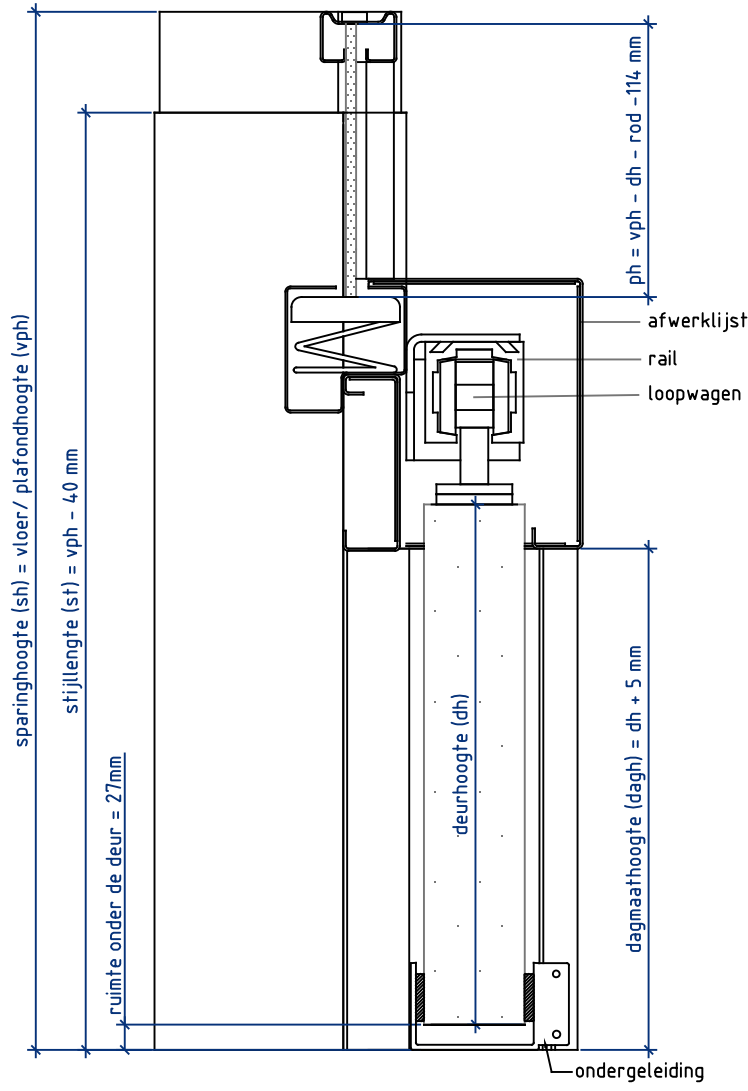
Doorsnede CC
