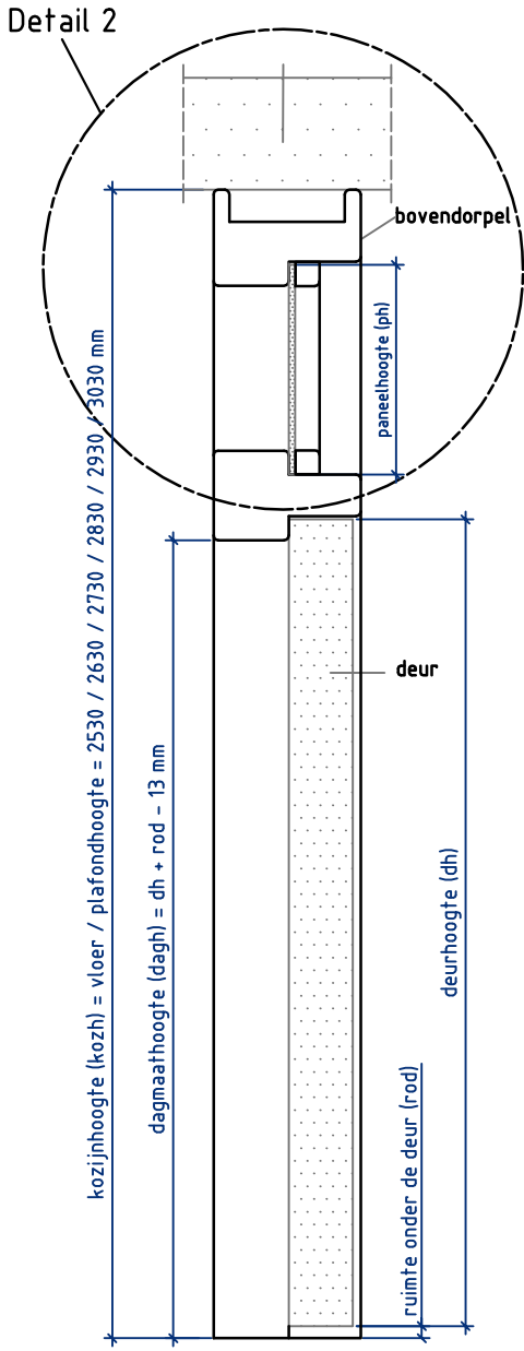
Doorsnede BB
