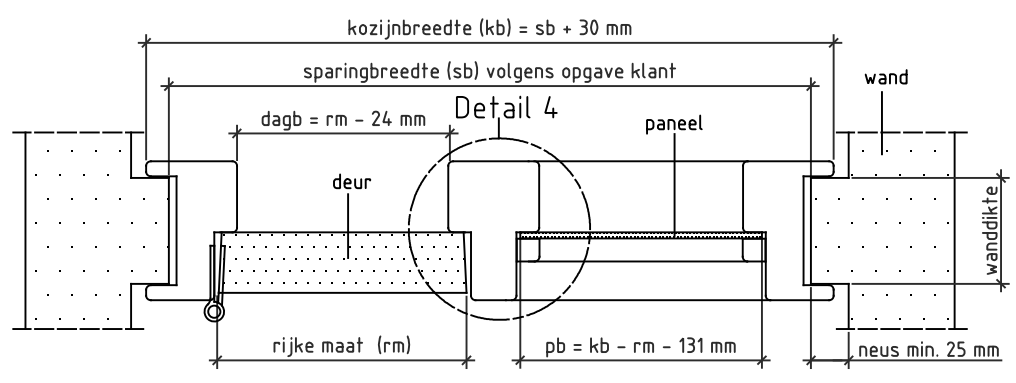
Doorsnede AA
