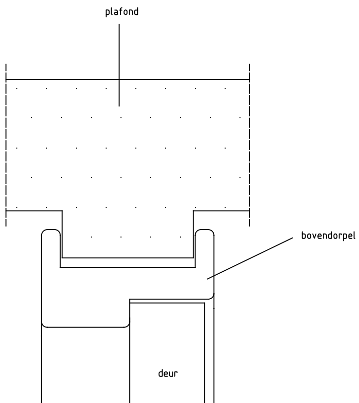
Detail 2: bovendorpel
