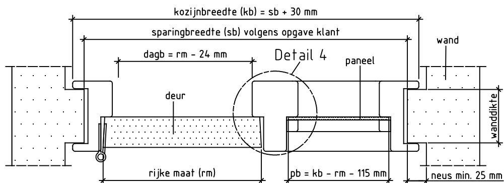
Doorsnede AA
