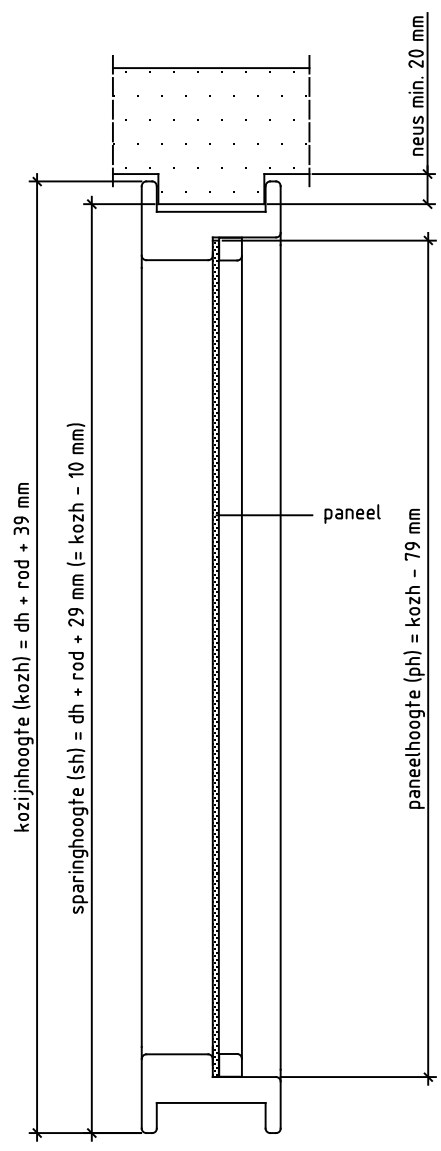
Doorsnede BB
