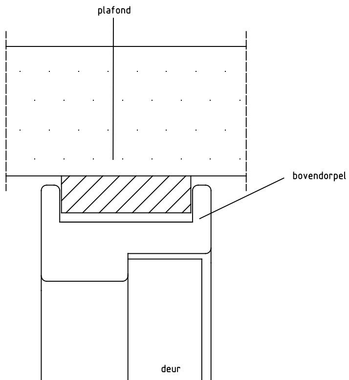
Detail 2: bovendorpel
