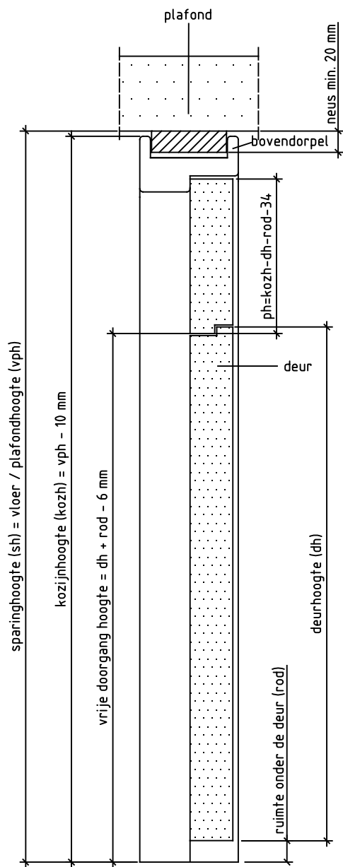
Doorsnede BB
