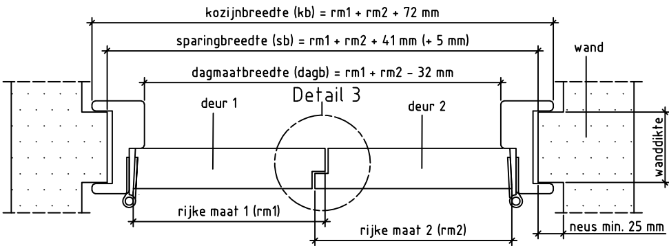
Doorsnede AA
