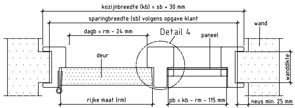
Doorsnede AA
