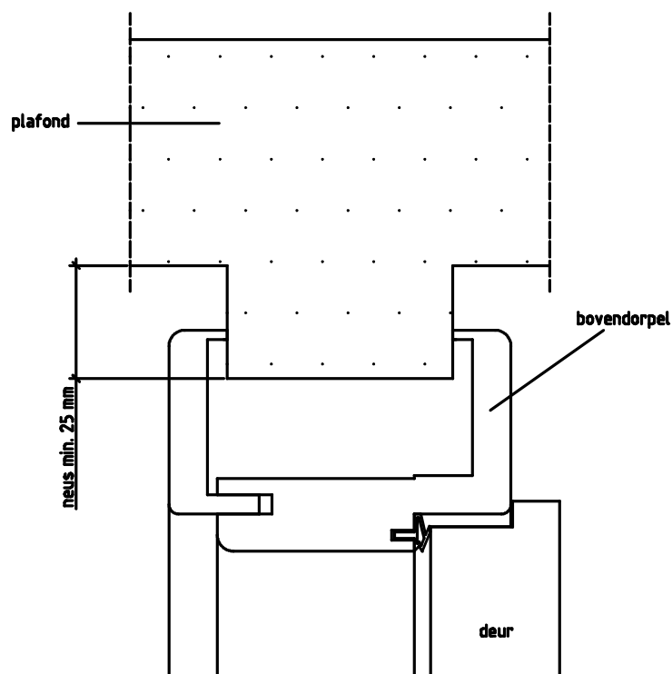
Detail 3: bovendorpel
