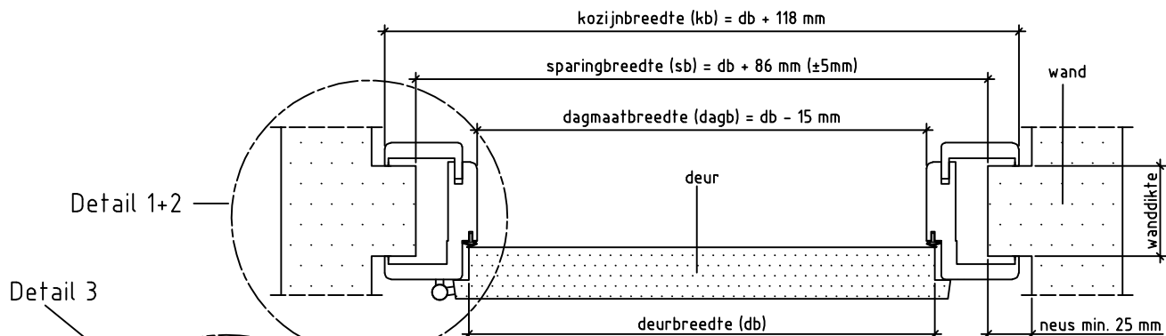
Doorsnede AA
