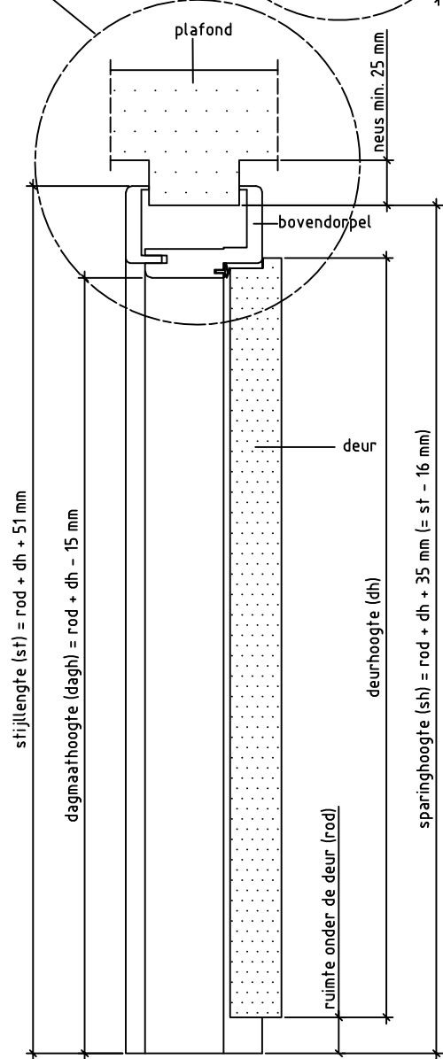
Doorsnede BB
