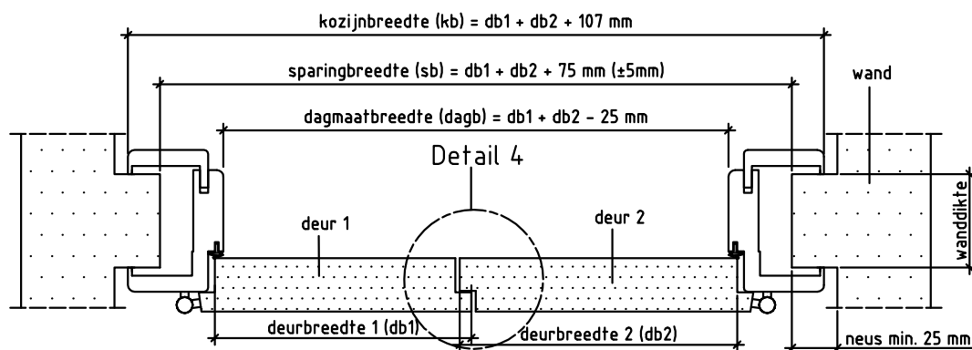
Doorsnede AA
