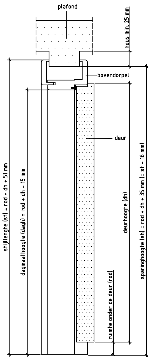
Doorsnede BB
