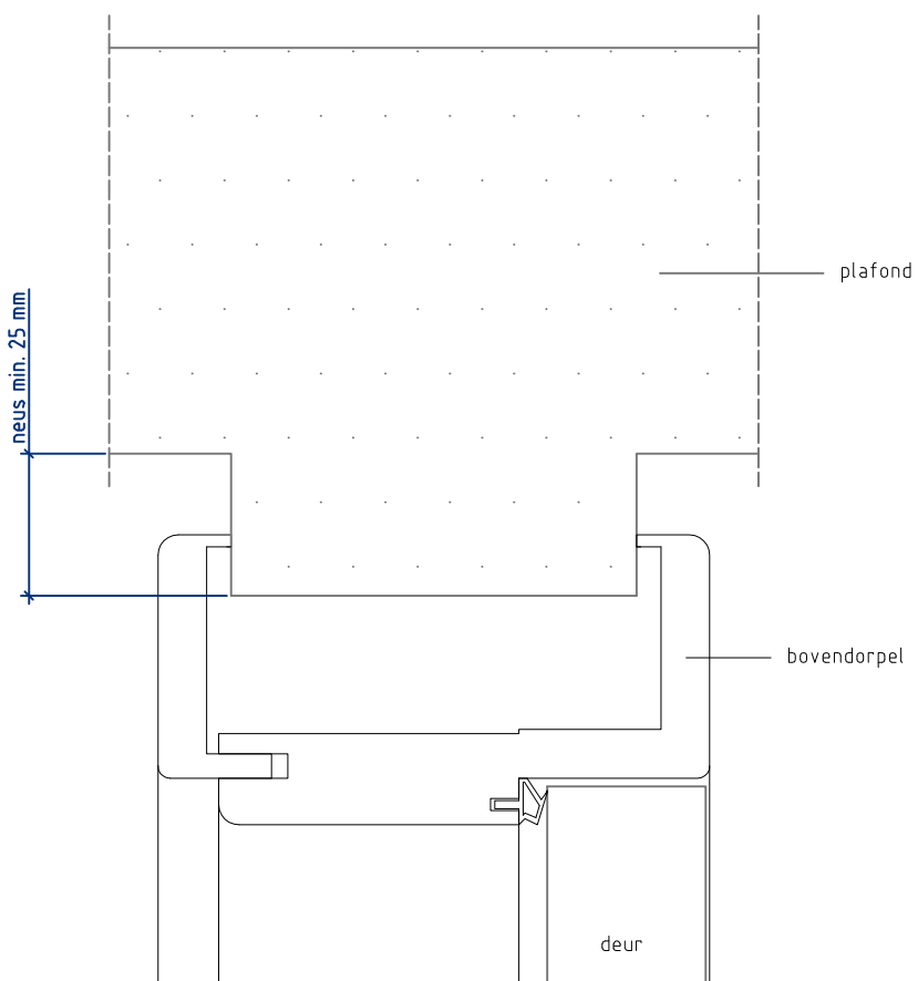
Detail 3: bovendorpel
