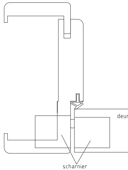
Optioneel verdekt scharnier
