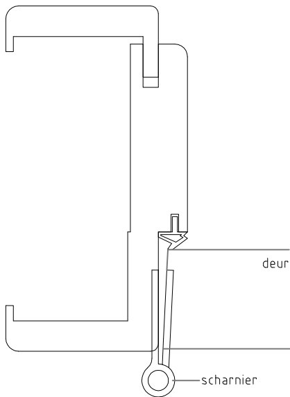
Detail 4: standaard scharnier
