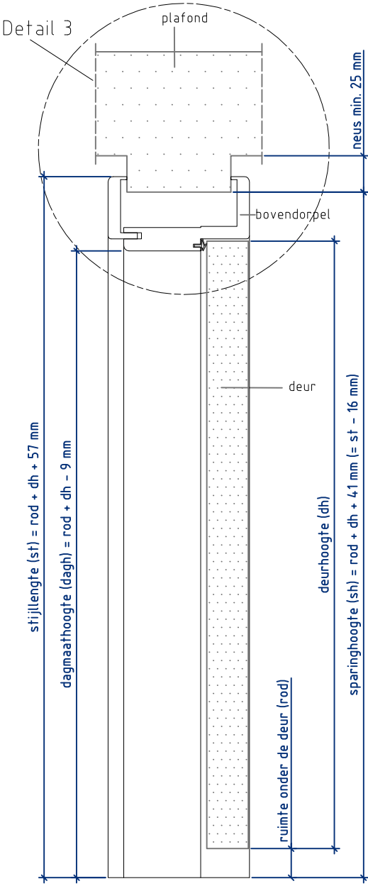
Doorsnede BB
