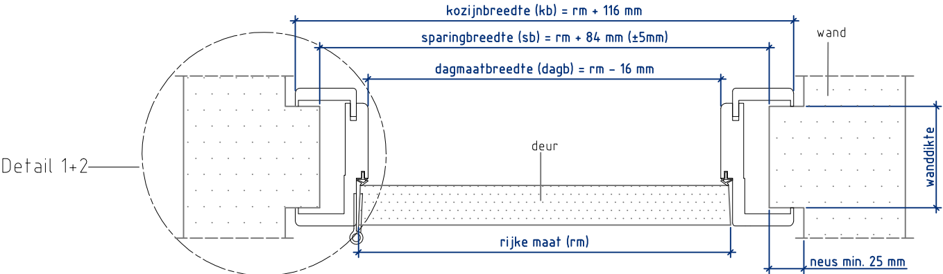
Doorsnede AA
