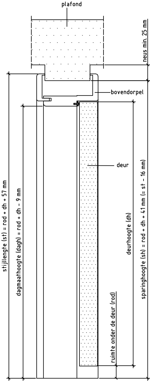
Doorsnede BB
