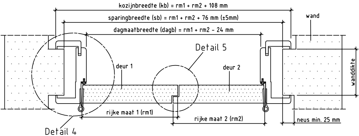
Doorsnede AA
