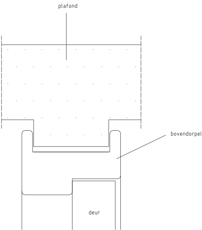
Detail 2: bovendorpel
