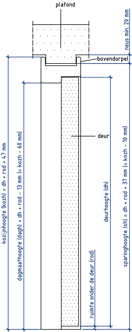
Doorsnede BB
