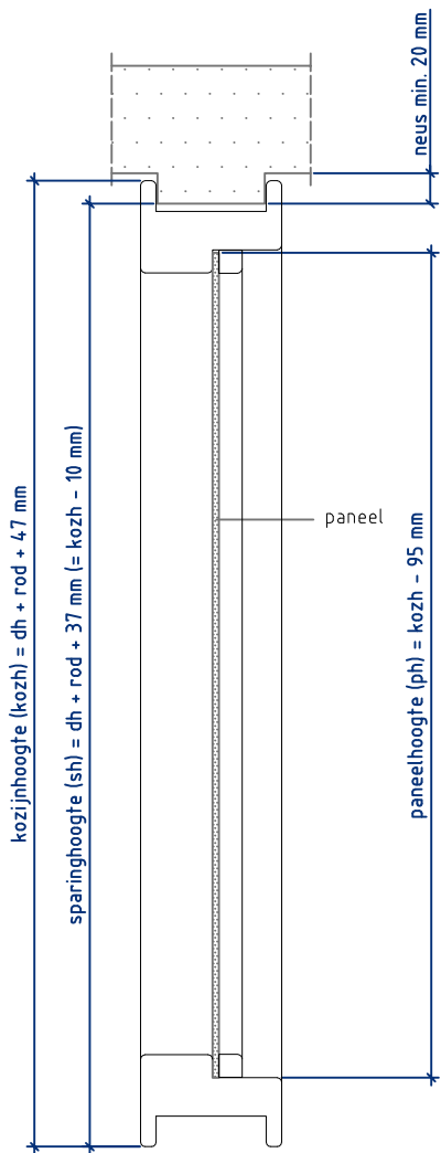
Doorsnede BB
