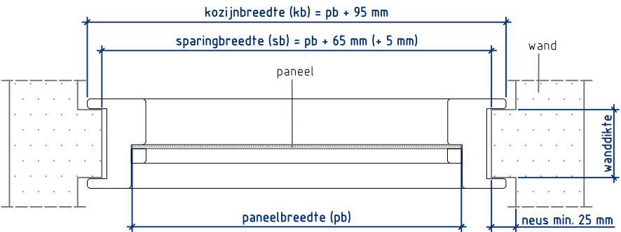
Doorsnede AA
