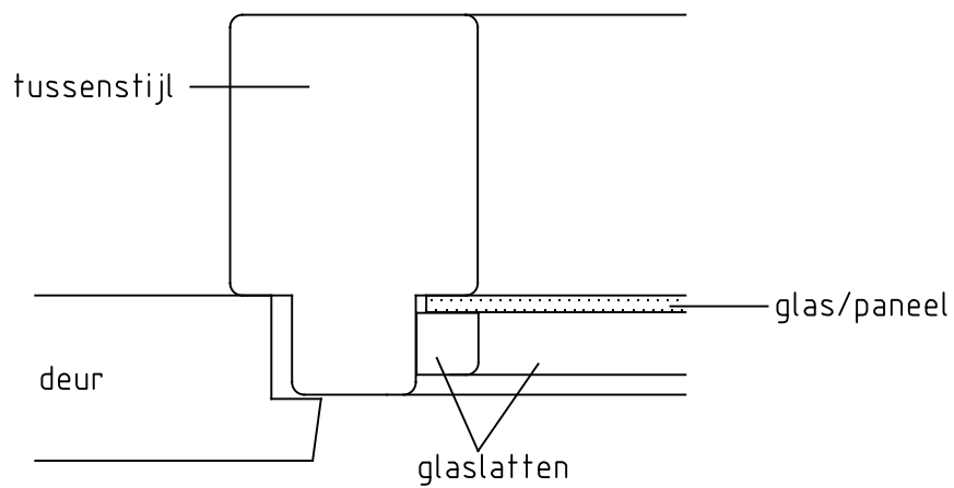
Detail 4: tussenstijl
