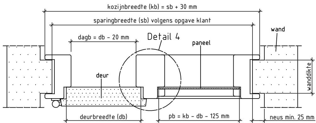
Doorsnede AA
