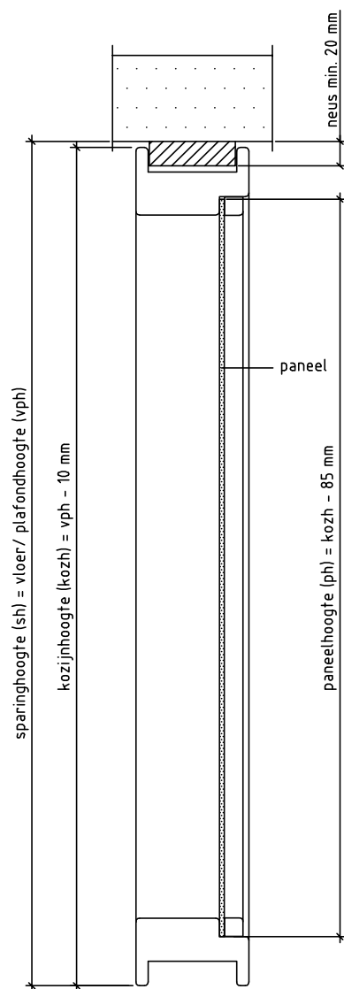
Doorsnede CC
