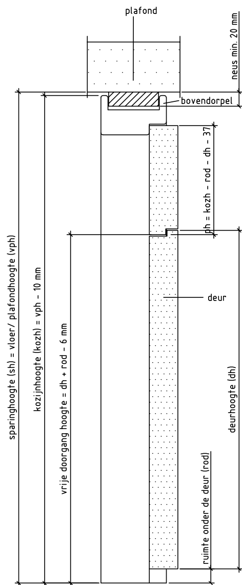
Doorsnede BB
