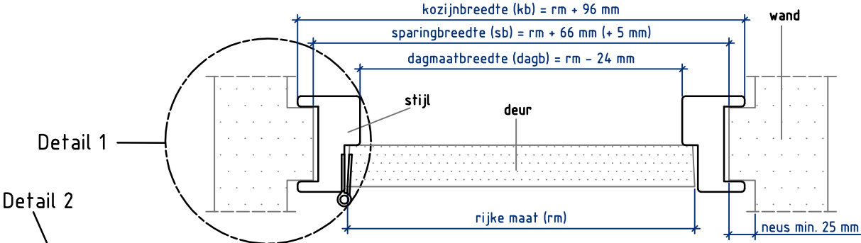
Doorsnede AA
