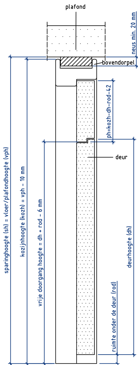
Doorsnede BB
