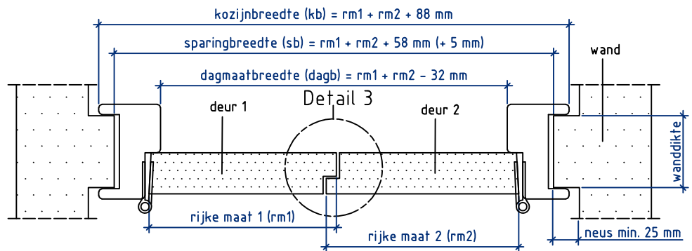
Doorsnede AA
